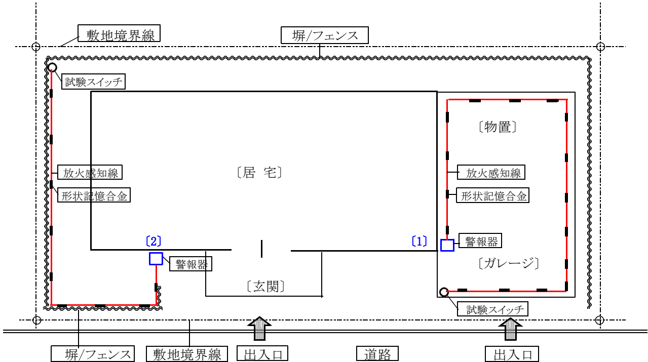
〔 配置 平面 図 〕
